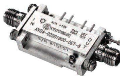
Рис. 8. Усилитель мощности AVG4-00101200-DET-8
