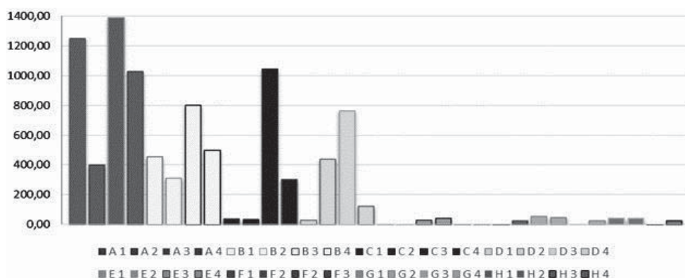
Рис.3. Распределение нефтяных углеводородов донных отложений
