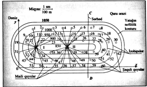
Şəkil 1. Birinci dəniz neft yatağının struktur xəritəsi
