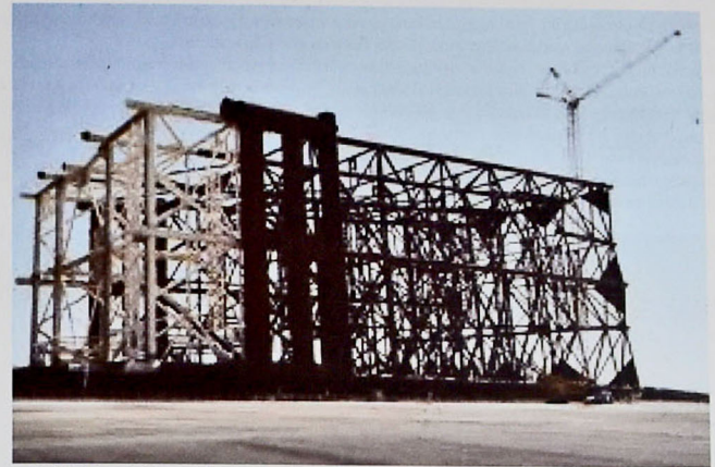
Şəkil 10. "Qarabağ" yatağında qoyulacaq platformanın dayaq bloku
