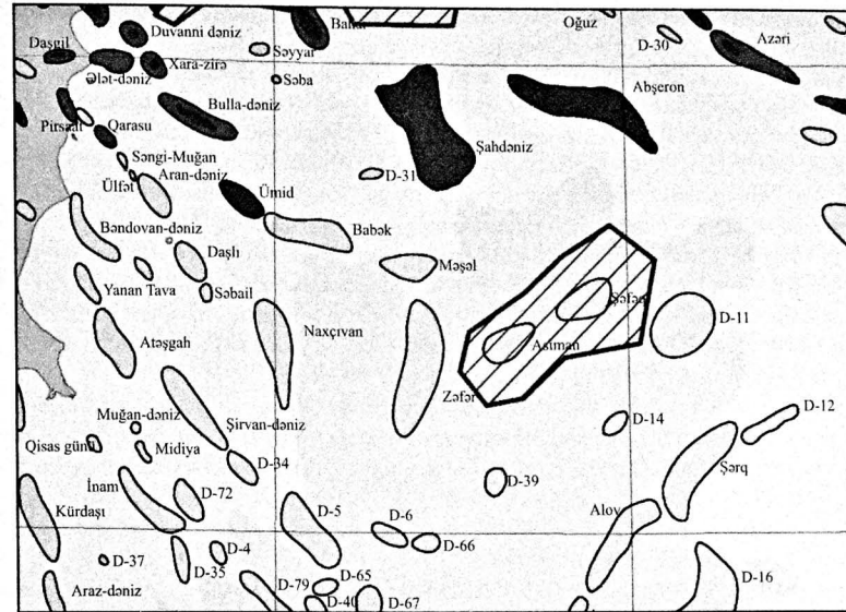
Şəkil 4. Şəfəq-Asiman strukturlarının yerləşmə sxemi
