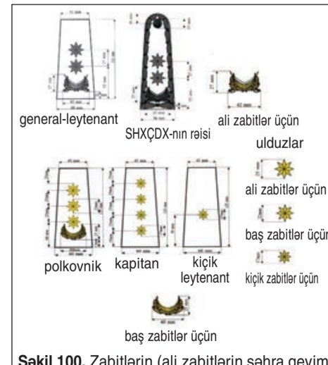
Şəkil 100. Zabitlərin (ali zabitlərin səhra geyim formasının) taxılıb-çıxarılan poqonlarının, onlarda yerləşdirilmiş ulduzlarnın və emblemlərin ölçüləri
