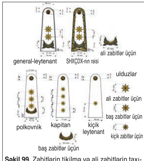
Şəkil 99. Zabitlərin tikilmə və ali zabitlərin taxılıb-çıxarılan poqonlarının (səhra-geyim formasından başqa), onlarda yerləşdirilmiş ulduzlarnın və emblemlərin ölçüləri
