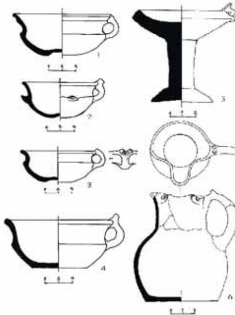
Şək. 2. 1-4-qulplu kasalar; 5-təkayaqlı vaza; 6-dolça
