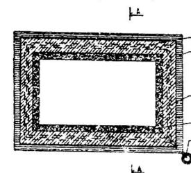
Рис. 4 Система обеспечения сухости заглубленной части сооружения
