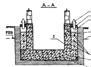
Рис. 2 Поперечное сечение А - А противофильтрационной системы
