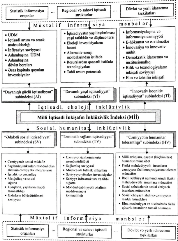
Şəkil 1. Milli iqtisadi inkişafın inküzivlik səviyyəsini formalaşdıran altindekslər və indikatorlar
