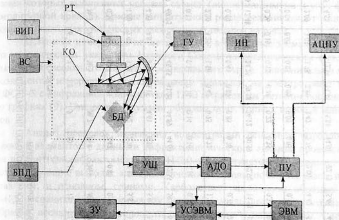
Рис. 1. ЗУ - загрузочное устройство для подачи проб в камеру образцов, ВС - вакуумная система, ГУ - гониометрическое устройство.
