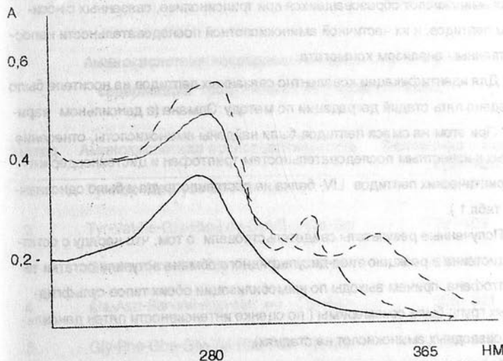
Рис. 1. Спектры поглощения исходного (—), модифицированного (---) и восстановленного (···) LIV-белка.
